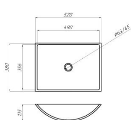
СФРК 520x380
