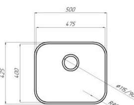
СФ 500
