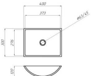
СФРК 400x300
