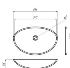
СФРК 566
