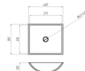
СФРК 400x350
