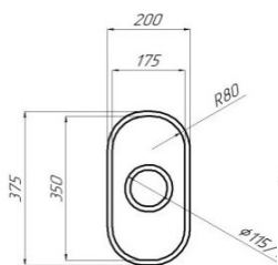
СФ 400
