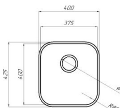
СФ 400
