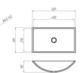
СФРК 520x300
