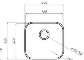
СФ 450
